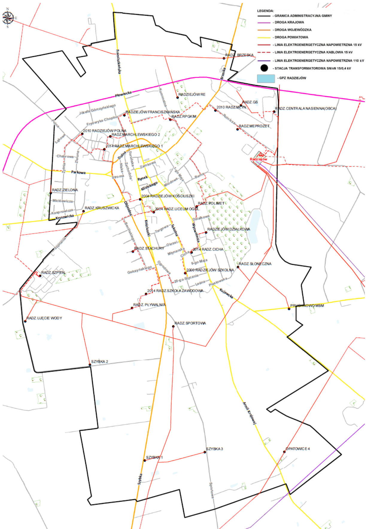
Ryc. 12. Przebieg linii elektroenergetycznych na terenie Miasta Radziejów
