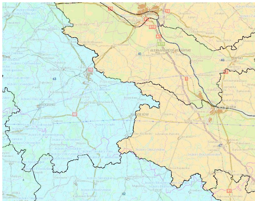
Ryc. 15. Położenie Miasta Radziejów na tle jednolitych części wód podziemnych
